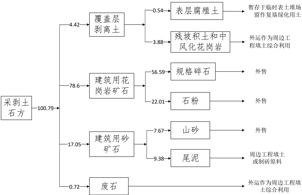
图 2-2 土石方平衡图 单位：万 t/a
