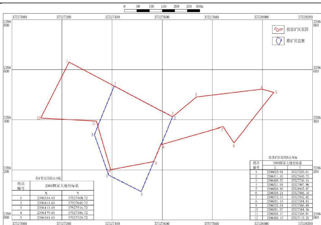
图2-1 原有矿区与本项目设置矿区范围叠合图
