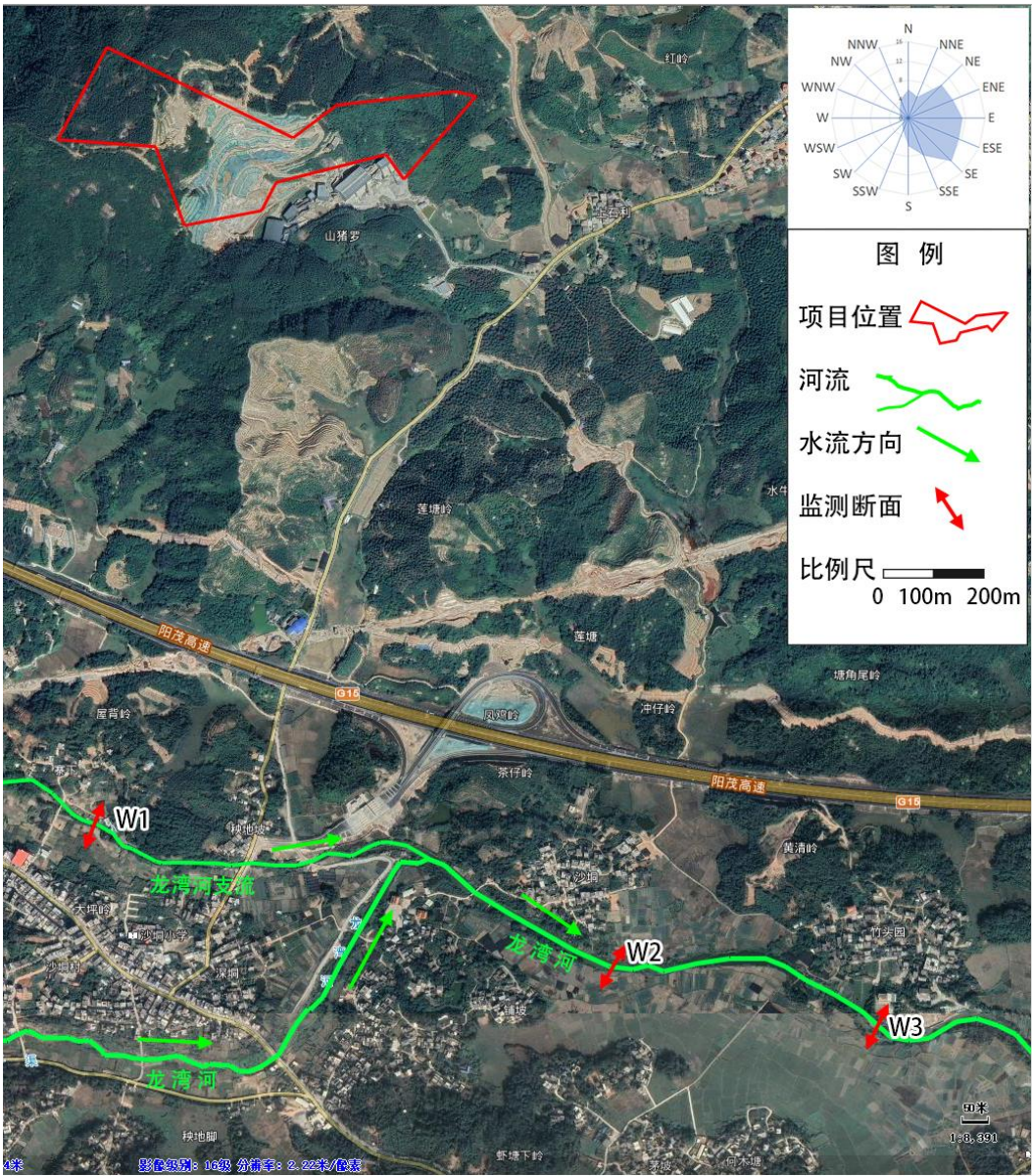
图 3-3 本项目附近地表水监测点位分布图
