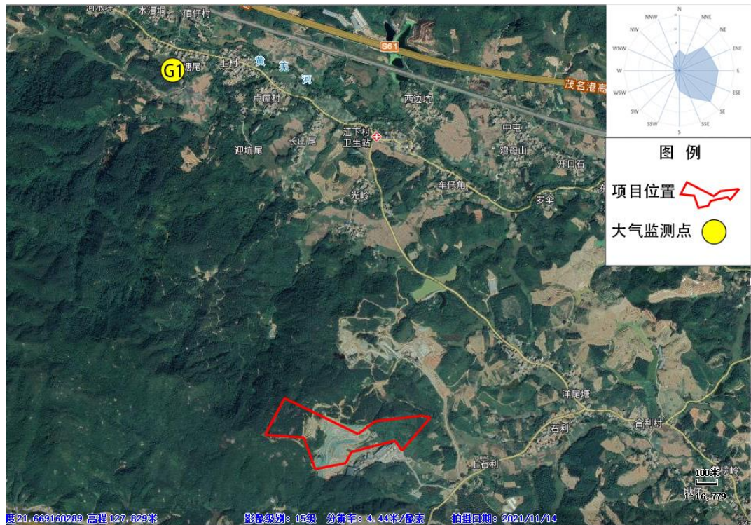
图 3-2 本项目大气环境监测点位分布图
