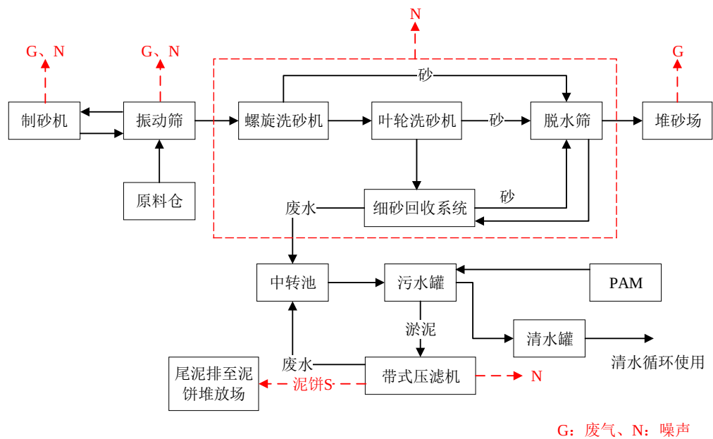
图 2-5 洗砂加工工艺流程及产污环节图
