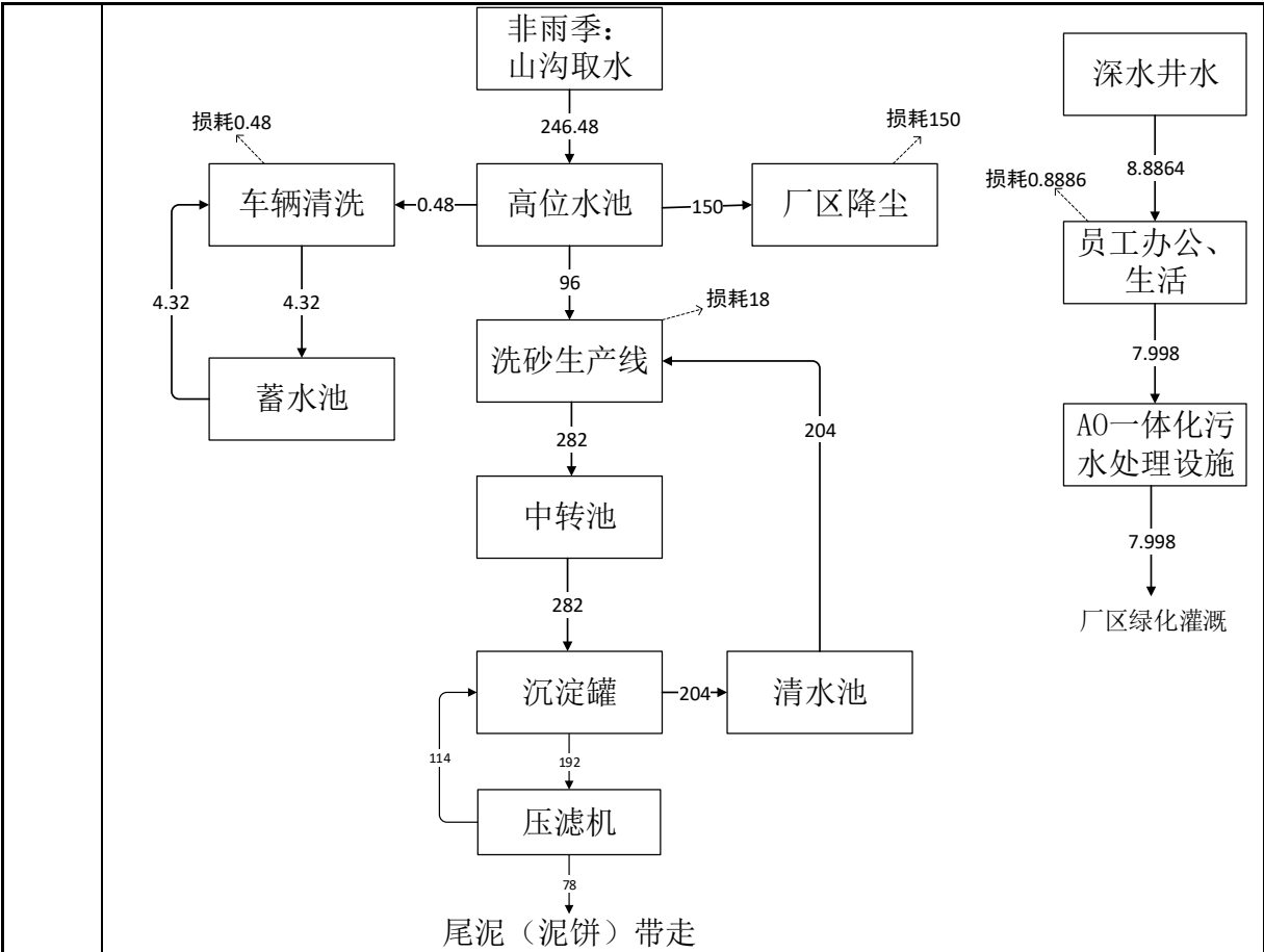
图 2-7 非雨季时水平衡图 单位：m³ /d
