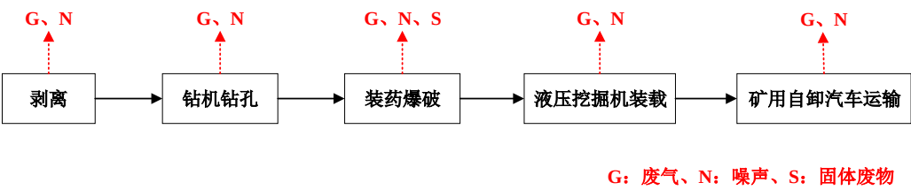
图 2-3 采剥工艺流程及产污环节图
