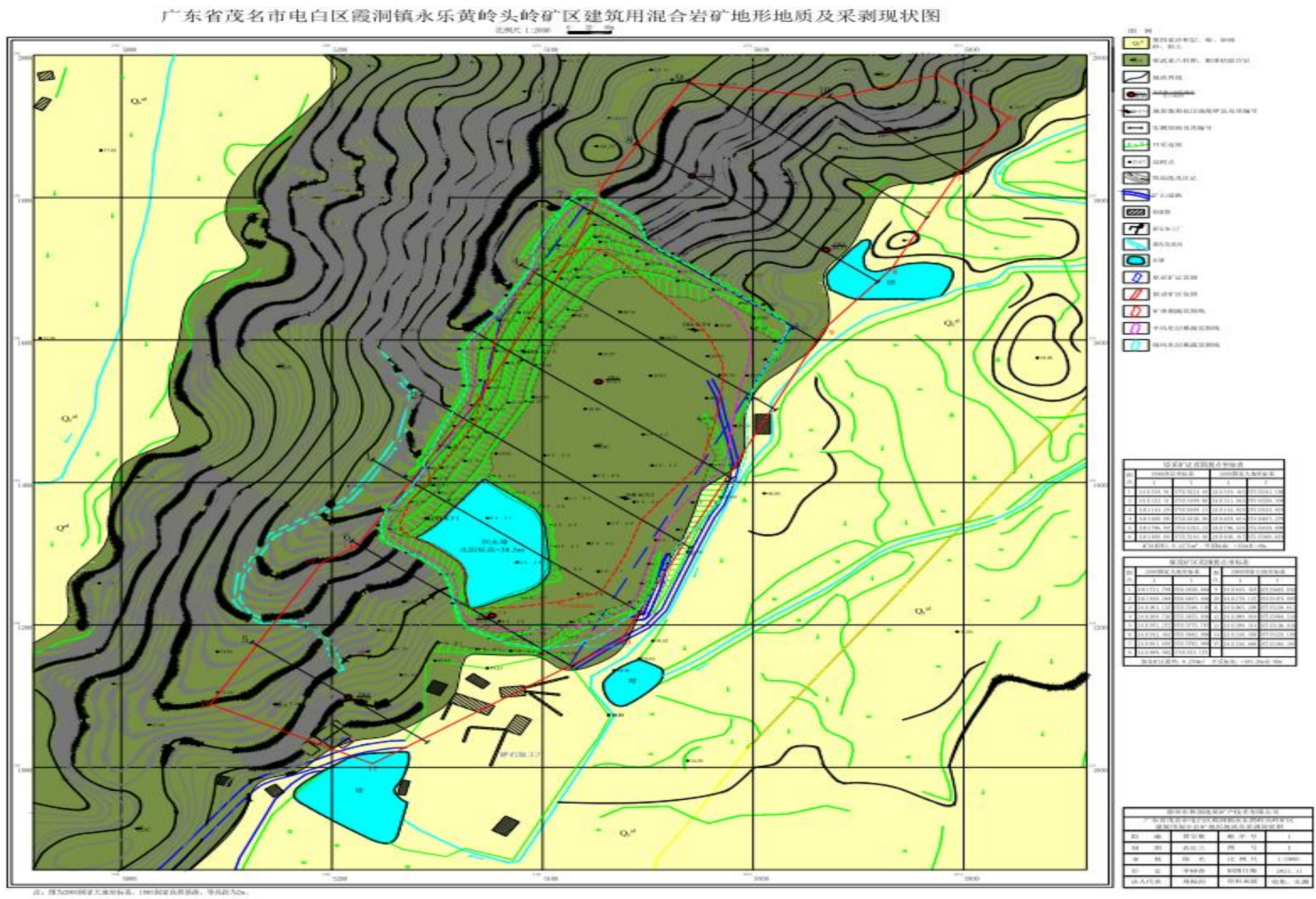
附图十四 永乐矿地形地质及采剥现状图
