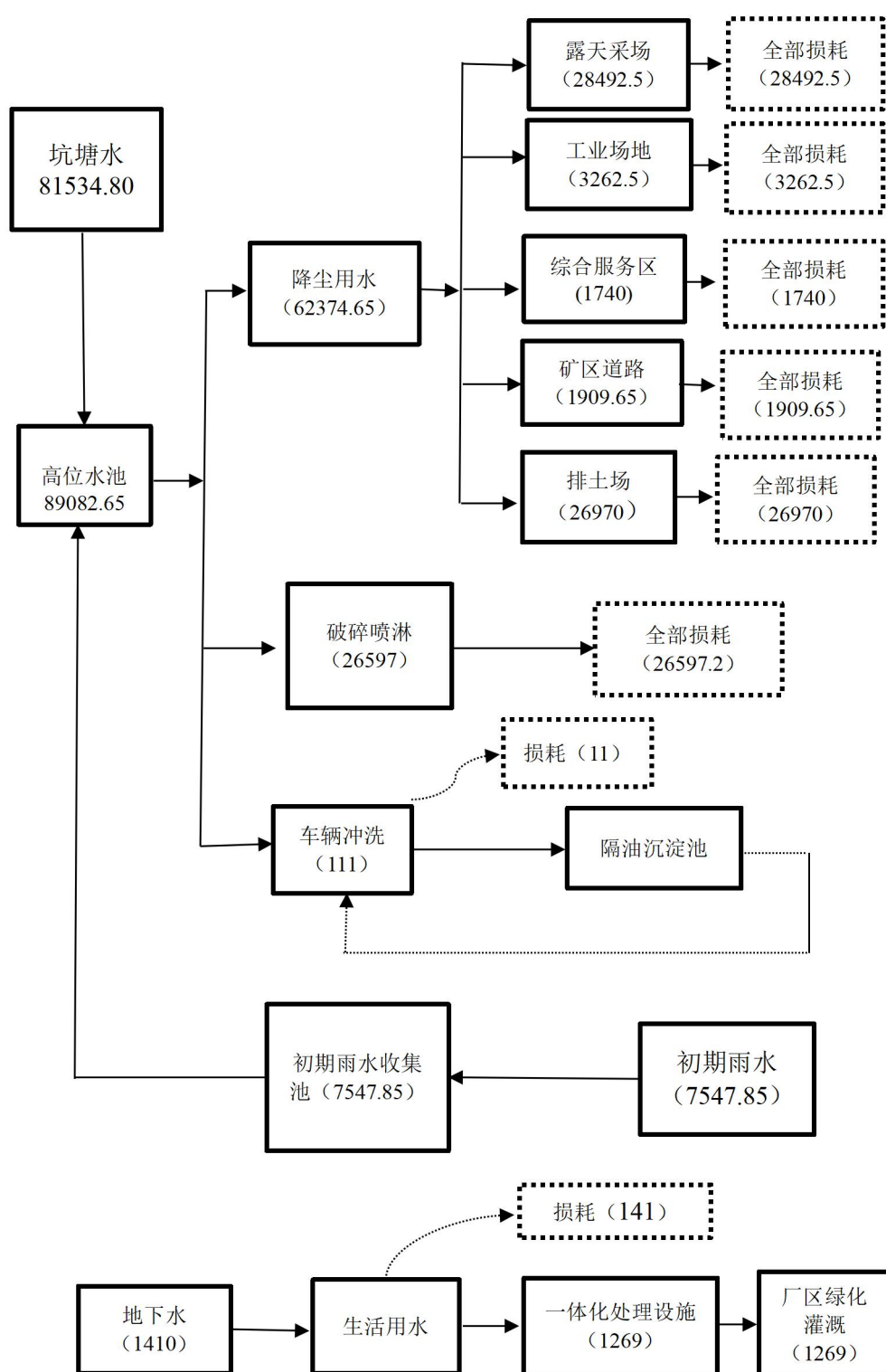
图 4-10 项目水平衡图 (单位 \text{m}^3/\text{a} )
