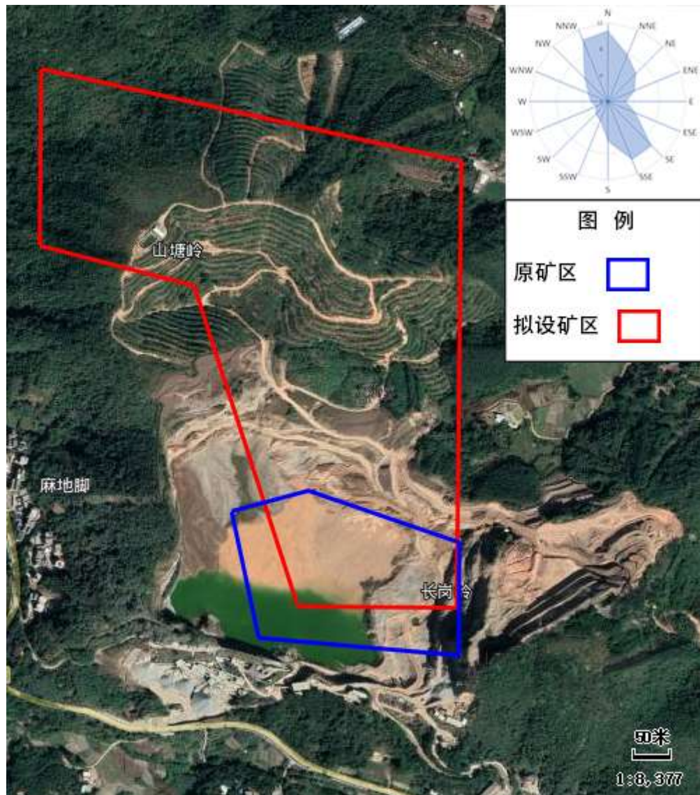
图2-1 原有矿区与本项目设置矿区范围叠合图
