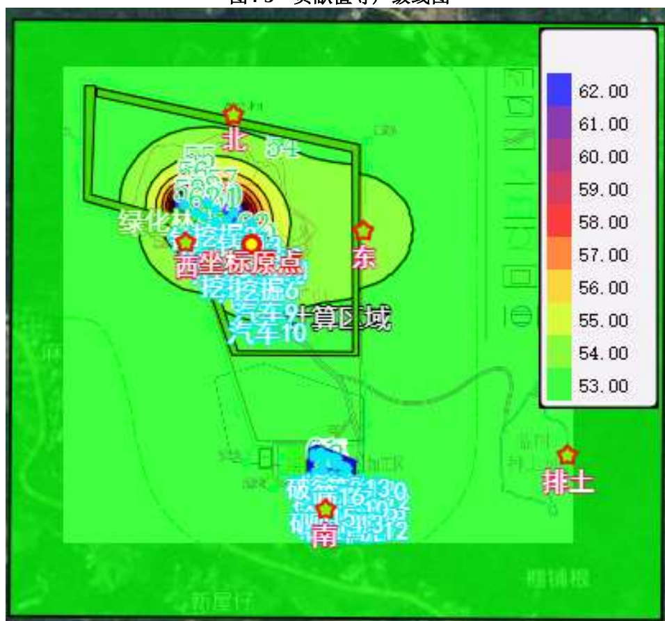
图4-4 预测值等声级线图
