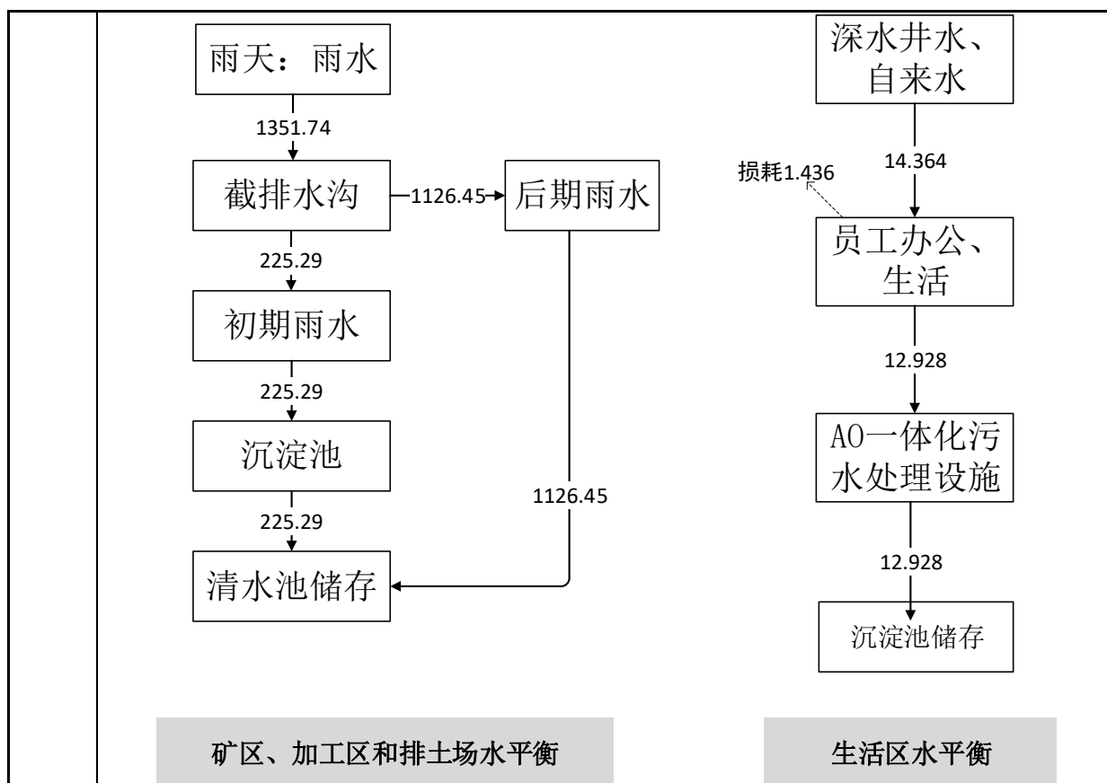
图 2-7 雨天时水平衡图 单位：m 3 /d
