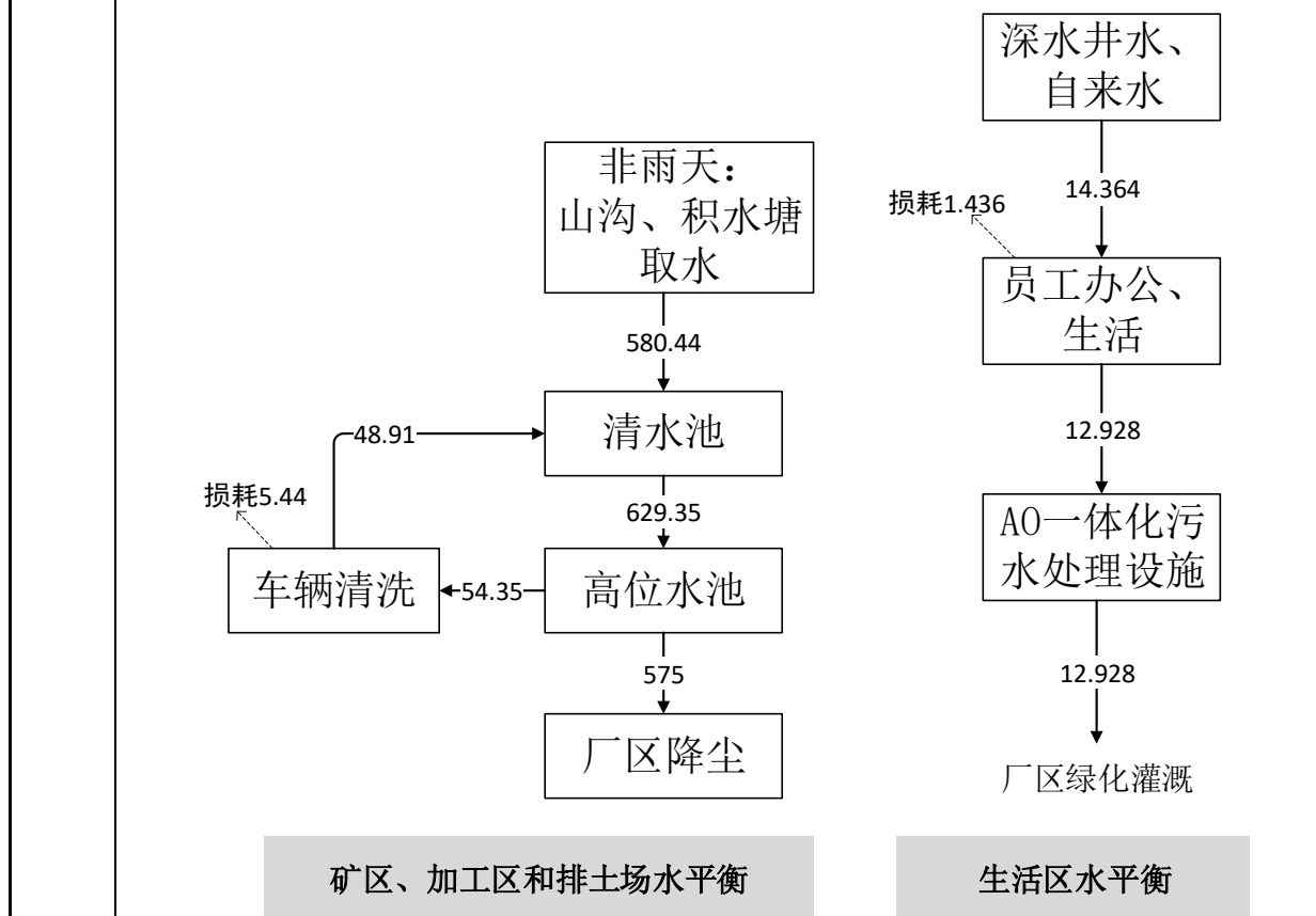
图 2-8 非雨天时水平衡图 单位：m 3 /d
