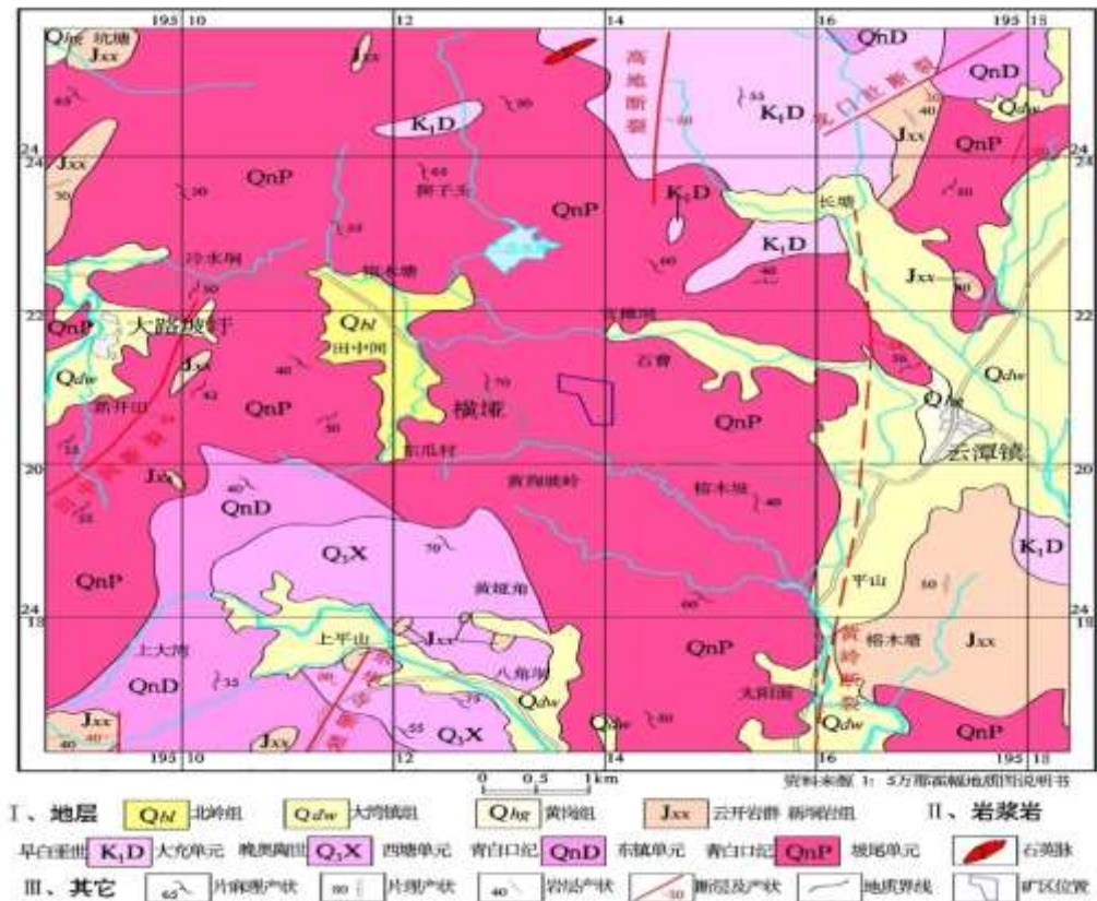
图 3-1 区域地质图(资料来源: 1:5 万那霍幅区域地质查报告)
