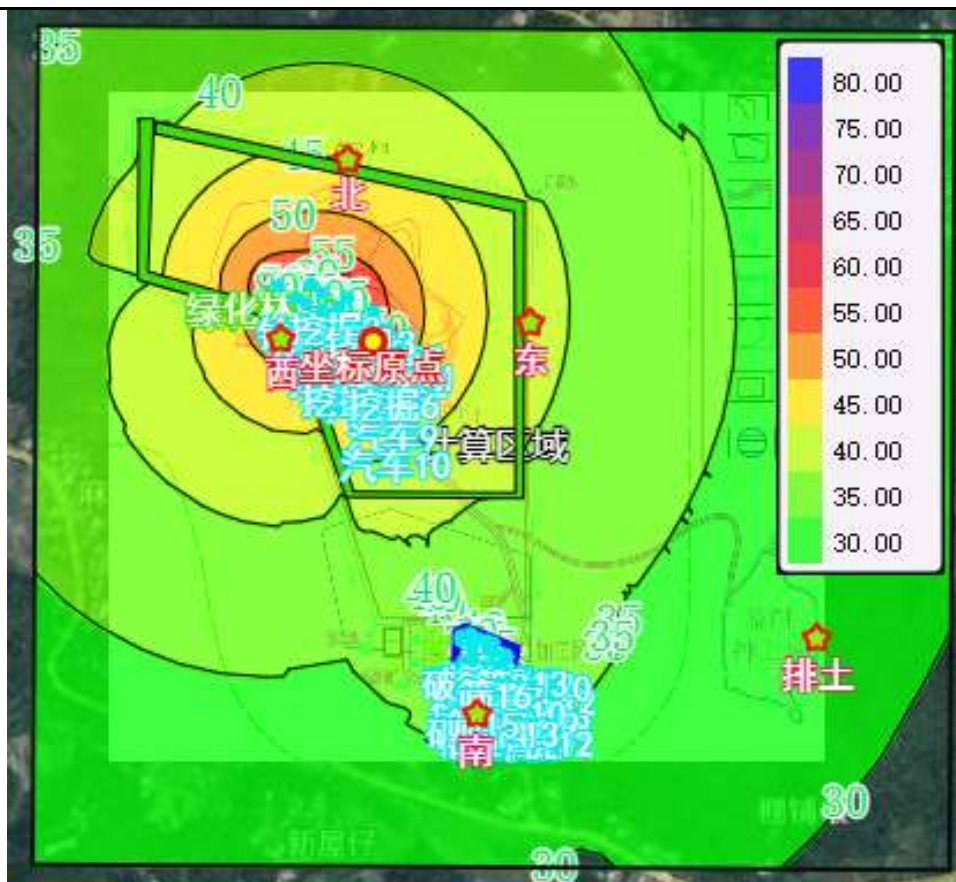
图4-3 贡献值等声级线图
