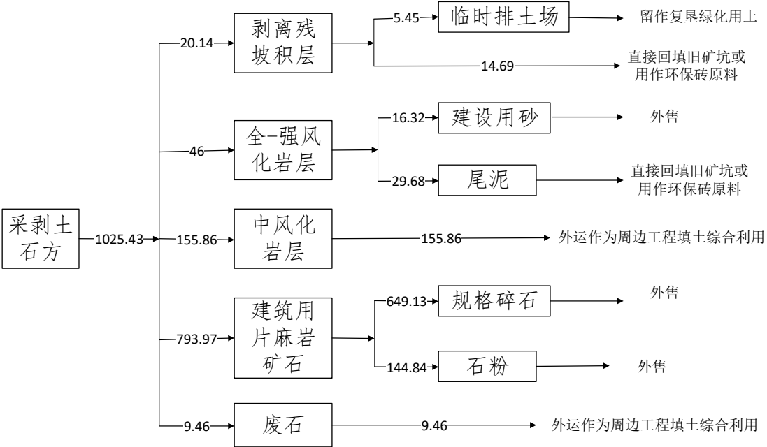
图 2-2 土石方平衡图 单位：万 t/a
