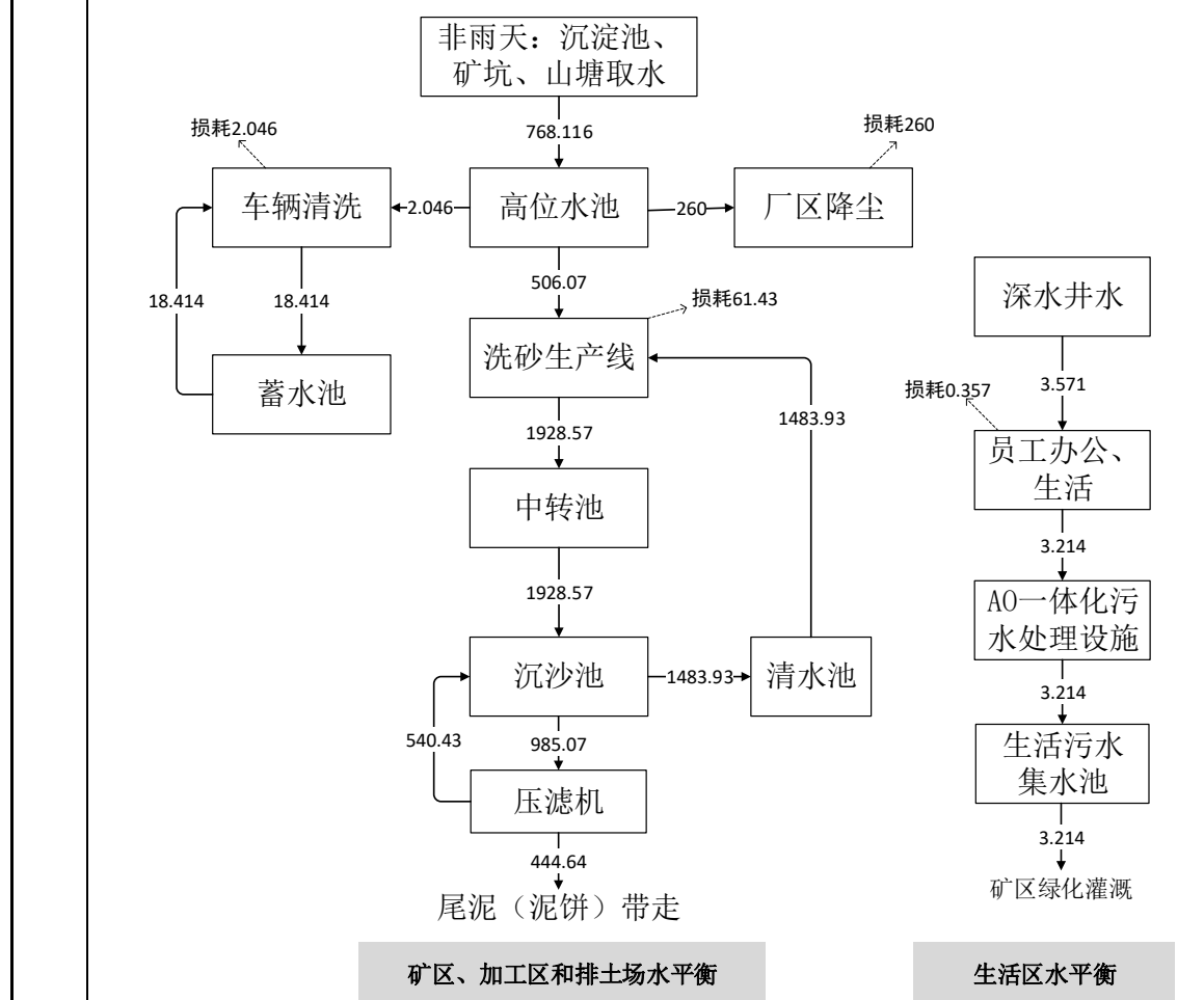
图 2-7 非雨天时水平衡图 单位: \text{m}^3/\text{d}
