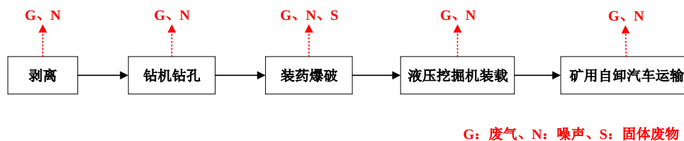
图 2-3 采剥工艺流程及产污环节图
