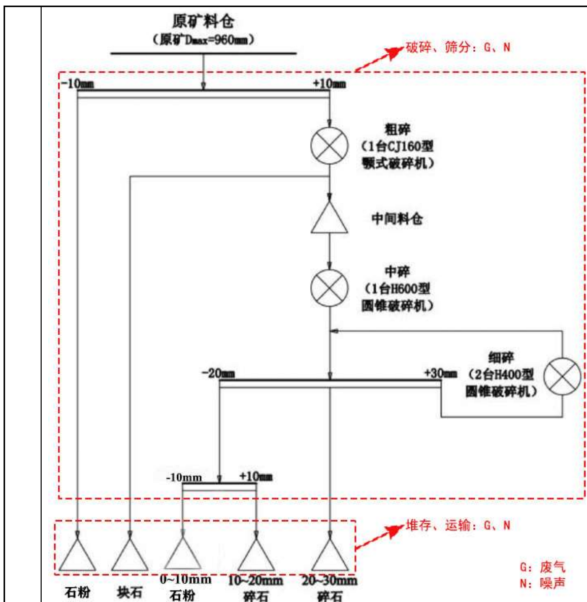
图 2-4 矿山破碎工艺流程图
