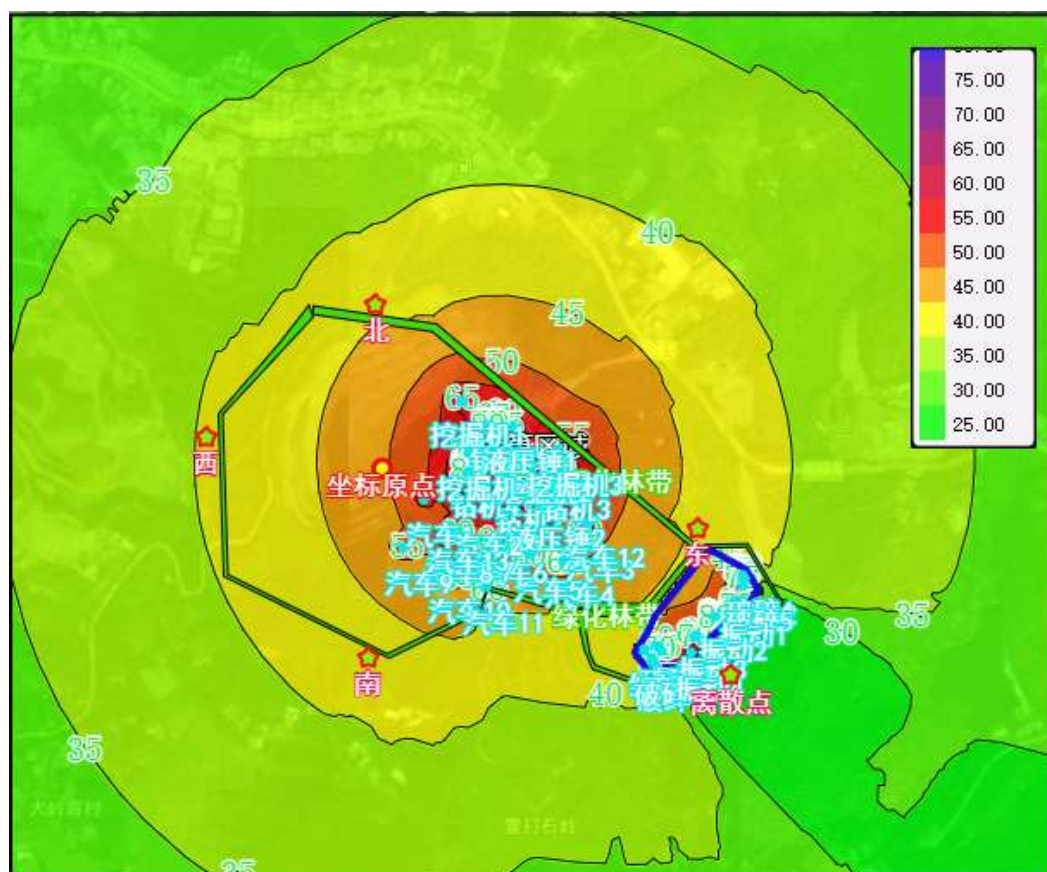
图4-3 贡献值等声级线图
