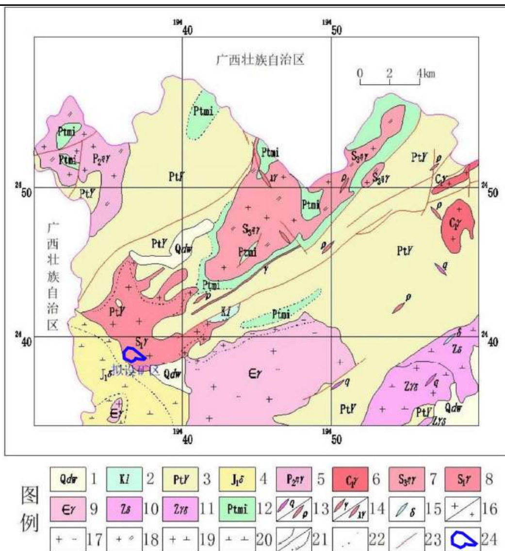
图 3-1 区域地质图（资料来源：1:20 万玉林幅地质图）
