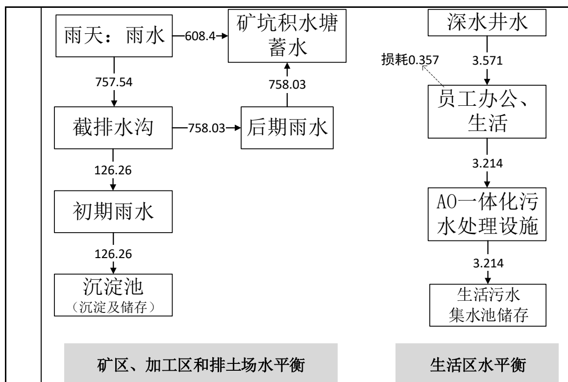
图 2-6 雨天时水平衡图 单位: \text{m}^3/\text{d}
