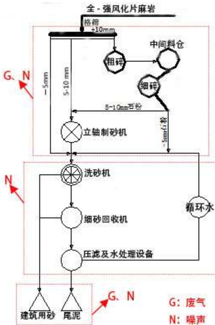
图 2-5 制砂加工工艺流程及产污环节图
